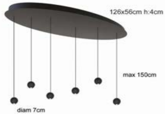
Ellips + 6x Pelota 6W 504lm
