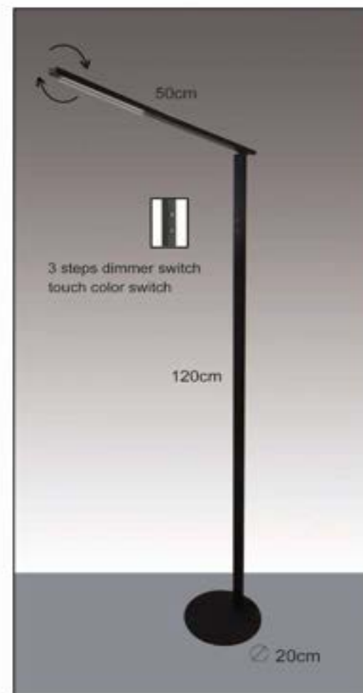
Pavi black 8W 600lm 3000K-6000K 93 81
