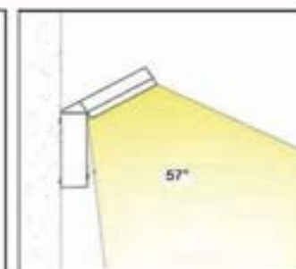
7014 wall black 12W 640lm 3000K IP54 93 163
