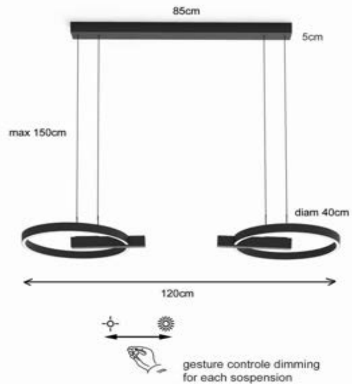
22 93 Arrow 2 sosp black 75W 3750lm 3000K dimmable
