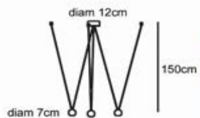
52 93 Pelota 3 black 3x6W 1512lm 2700K dimmable
